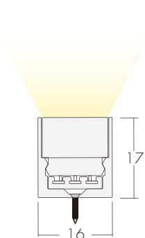
Carril superficie.
