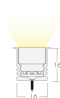
Carril empotrar.
